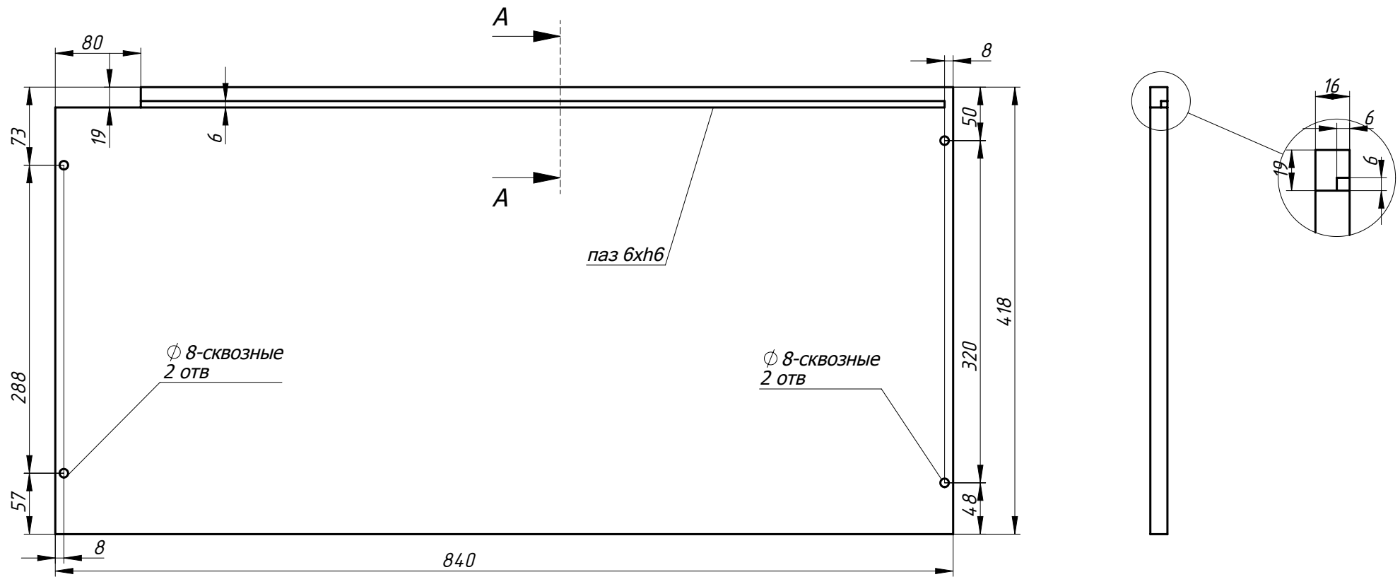
Пол шкафа-47
