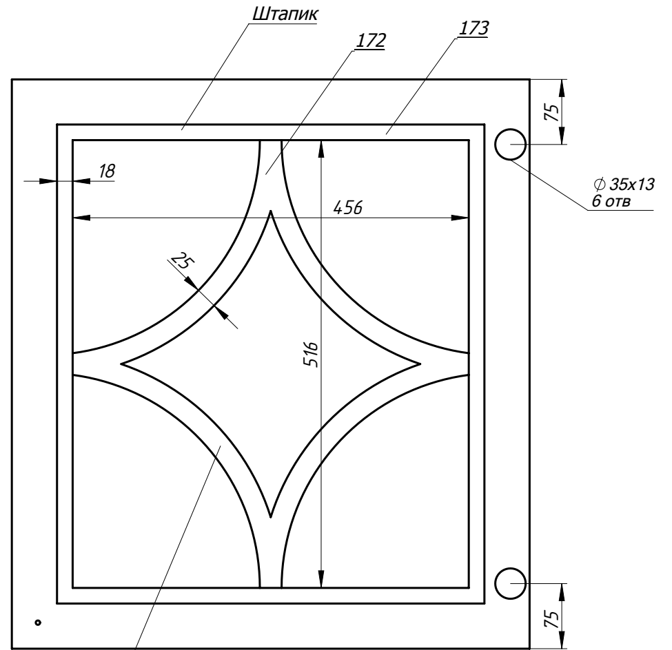
Внутренняя накладка
