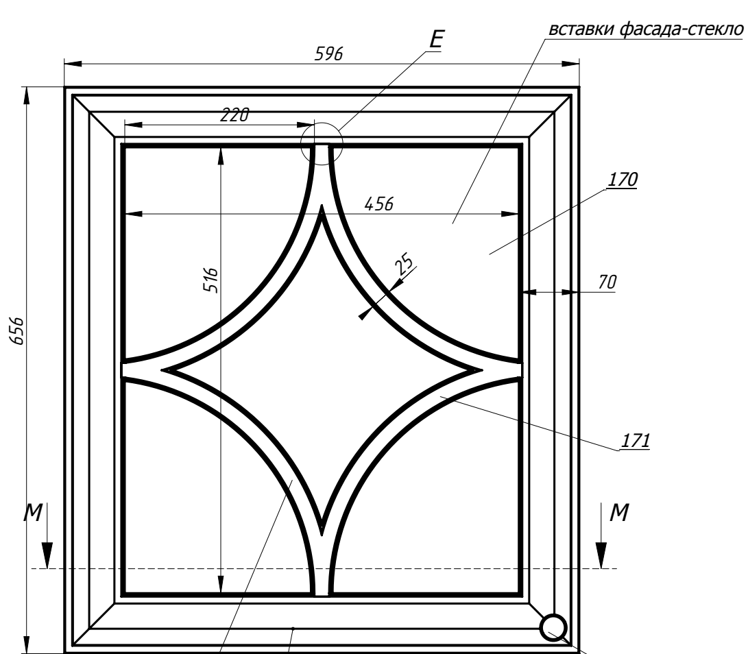
Передняя накладка
