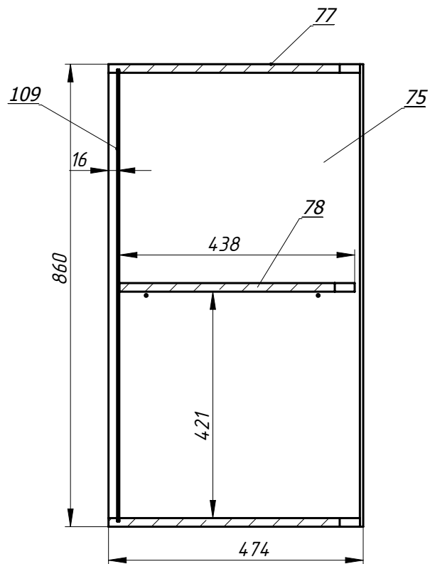
Корпус без фасадов Б-Б
